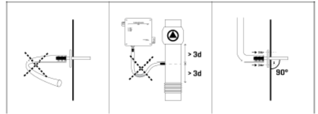
Rys. 3: Zalecenia montażowe
