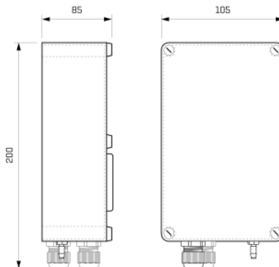
Rys. 1: Wymiary urządzenia w mm
